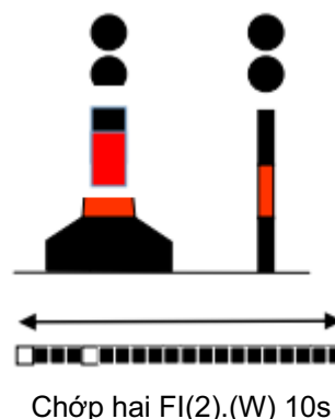
Hình 21: Báo vật chướng ngại hoặc vị trí nguy hiểm bên phía trái luồng tàu chạy (B2.2)
