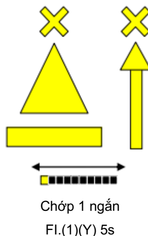
Hình 24: Phao giới hạn vùng nước phía bên trái luồng tàu chạy (B4.2)
