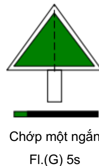
Hình 21: Báo vật chướng ngại hoặc vị trí nguy hiểm bên phía trái luồng tàu chạy (B2.2)
