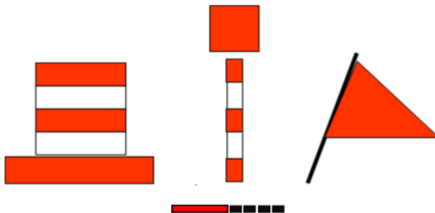
Hình 3: Phao chỉ vị trí giới hạn của luồng tàu sông đi cạnh luồng tàu biển, đặt bên phải luồng tàu sông (A.2.1)
